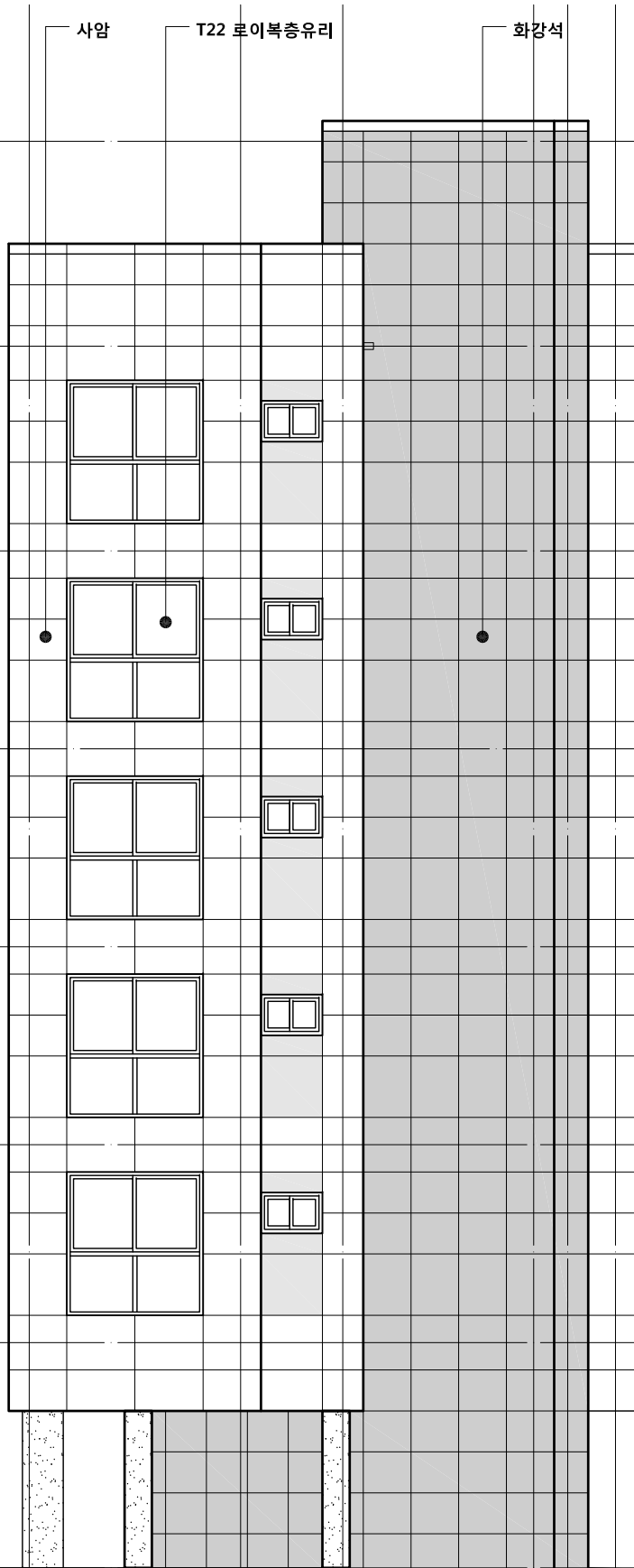
1 좌측면도 A - SCALE : 1/100
